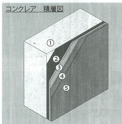
軽量かつ丈夫な構造
